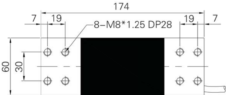
俯视（Top View）
